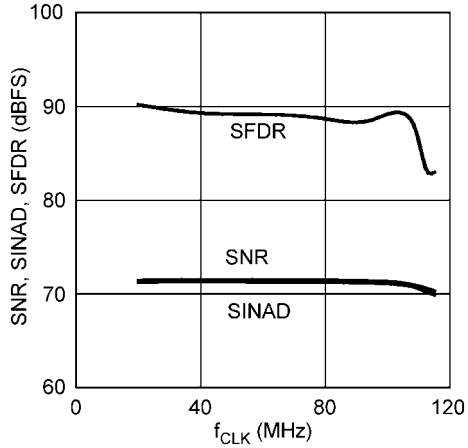
SNR, SINAD, SFDR vs. f_{CLK}
